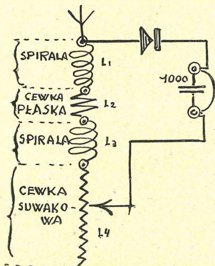
SZEMAT IDEOWY
