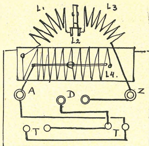
SZEMAT MONTAŻOWY.
