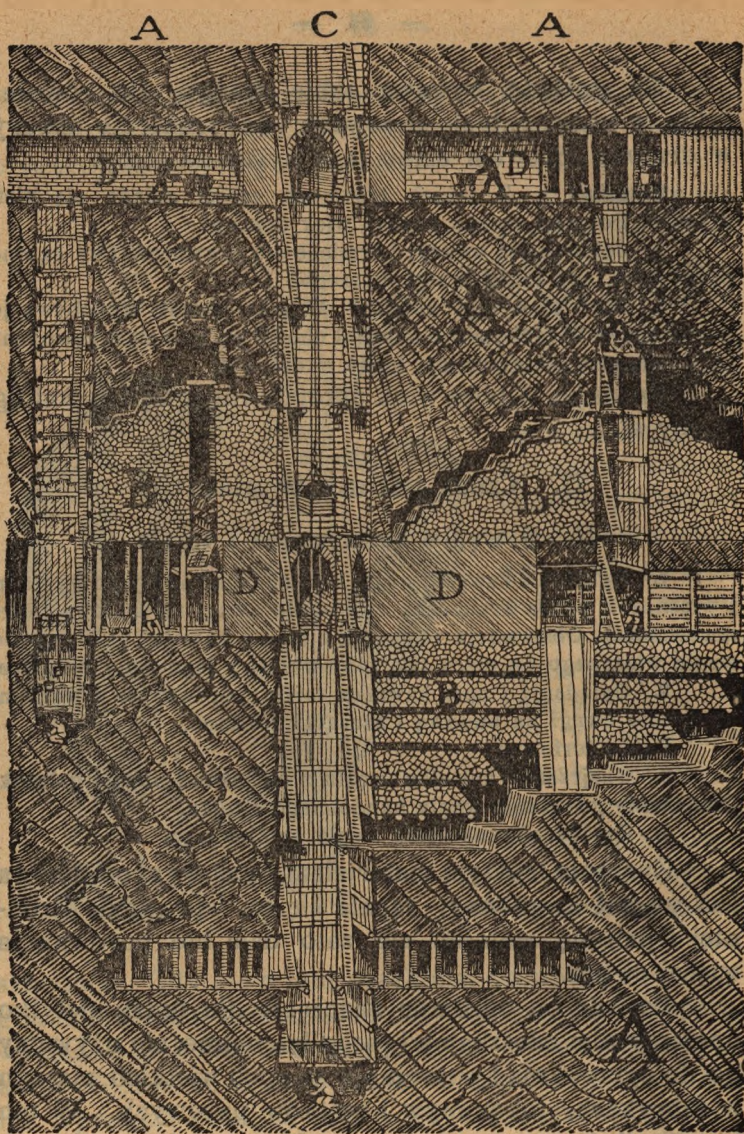
Wnętrze kopalni węgla. A — pokłady węgla. B — puste przestrzenie po wydobyciu węgla, zapełnione piaskiem albo gruzem. C — szysz pionowy. D — chodnik poziomy.
